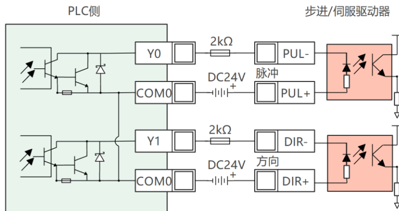
图 3-4 高速脉冲输出接线图
