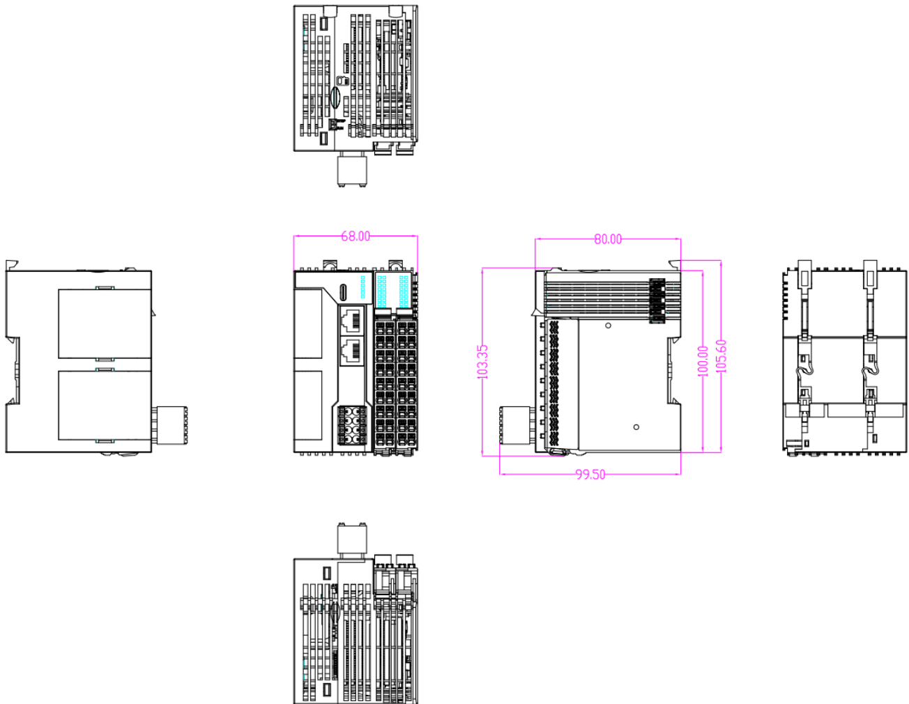
图 4-3 S304/S306/S308型号外观尺寸(单位: mm)
