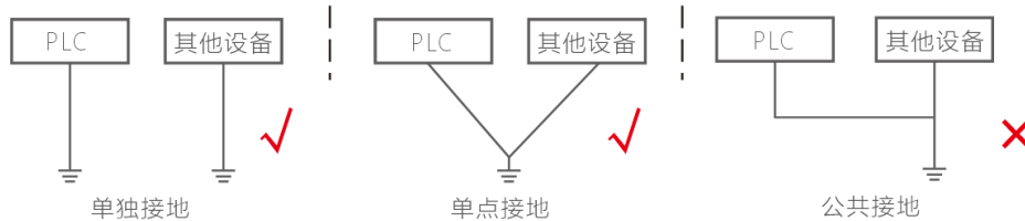
图 1-1 接地类型图
