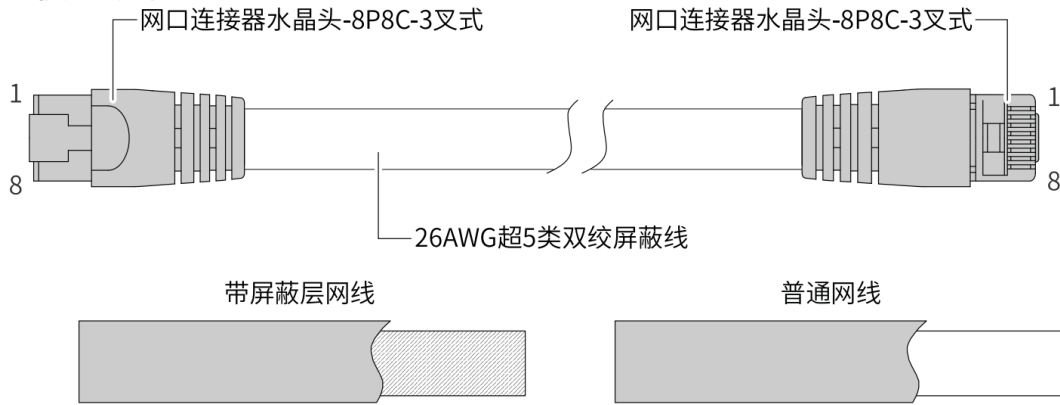
图 5-2 以太网线缆
