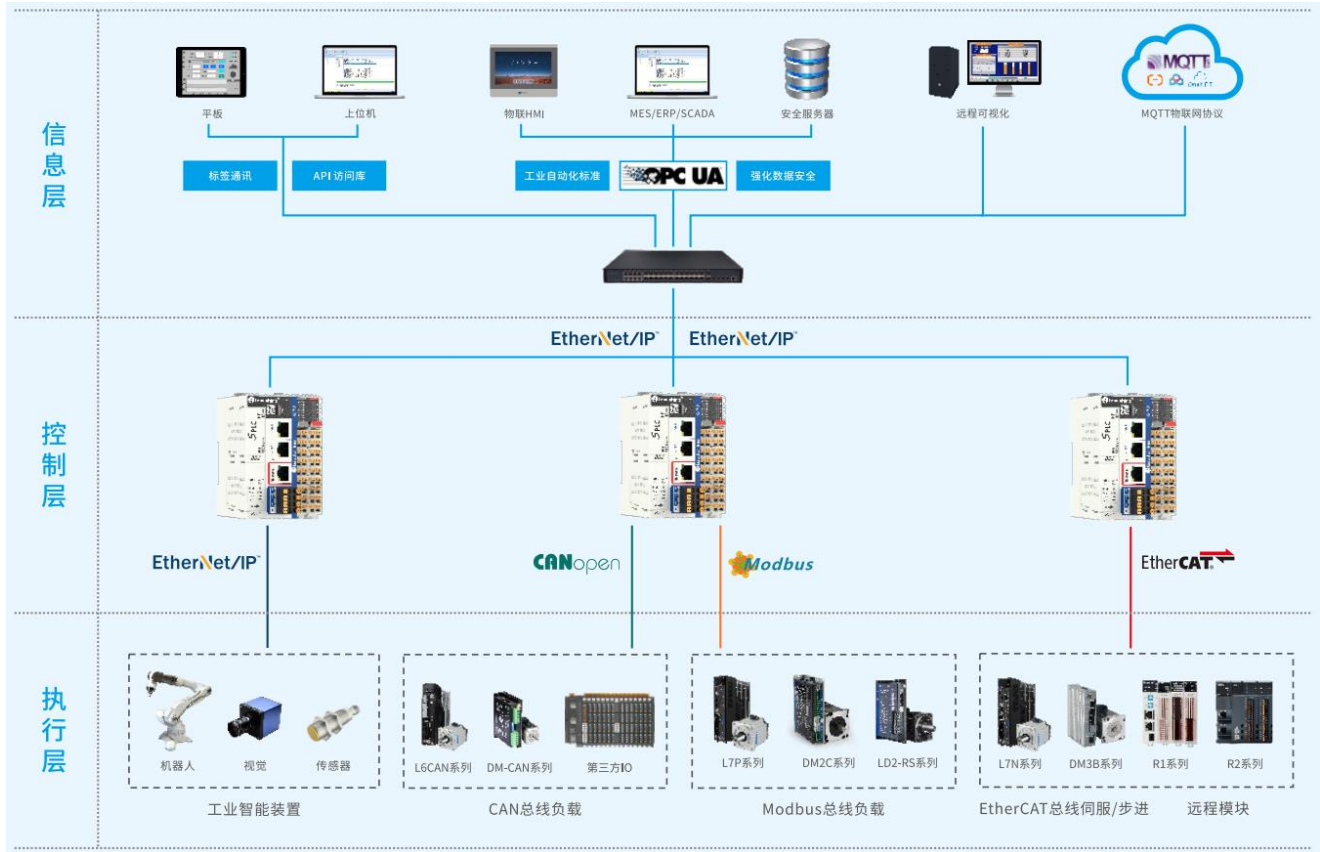
图 5-1 灵活组网
